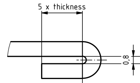
Detail B ( 4 : 1 )
