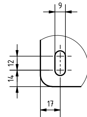
Detail C ( 1 : 2 )
